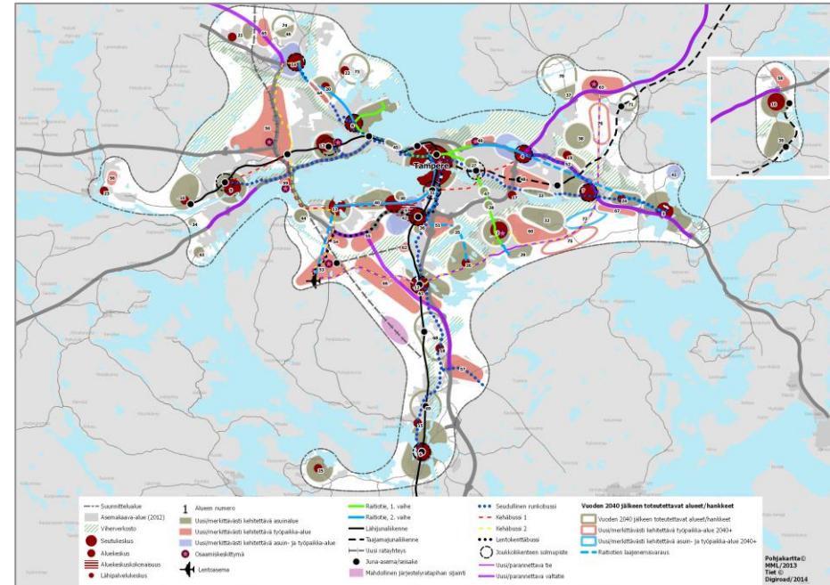
Rakennesuunnitelma vuoteen 2040
